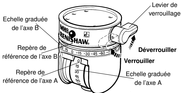
Figure 4 – Fonctionnement du levier de verrouillage
